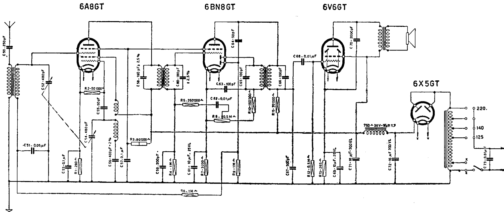
LA VOCE DEL PADRONE. — Mod. « 475 Super-Reflex ». — Telaio 75,1. — MF: 465 kHz. — Produzione: 1942-45.
